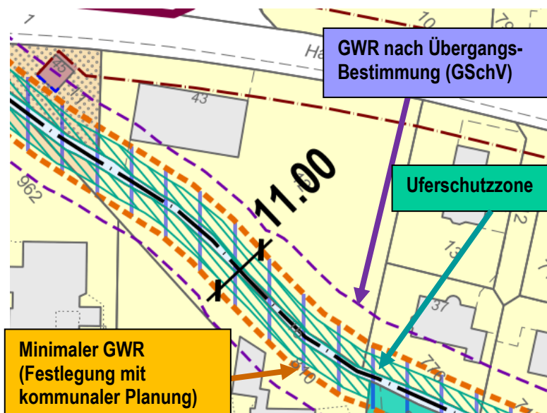
Auszug Entwurf Gewässerraumplan
